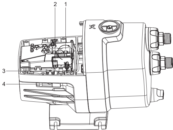
Conexión de la entrada externa
