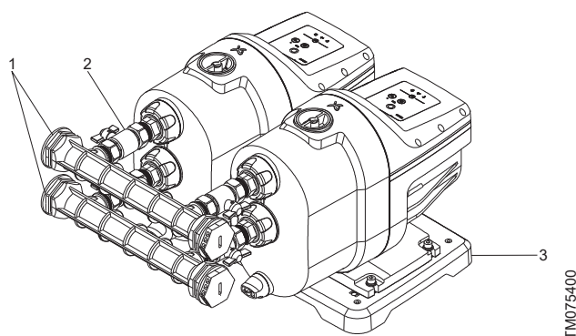
Sistema de aumento de presión doble SCALA1
