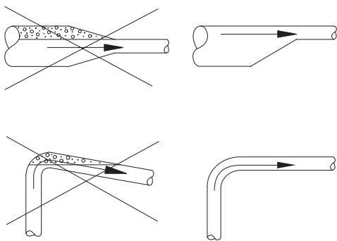
Instalación recomendada de las tuberías para evitar las pérdidas por fricción y las bolsas de aire
