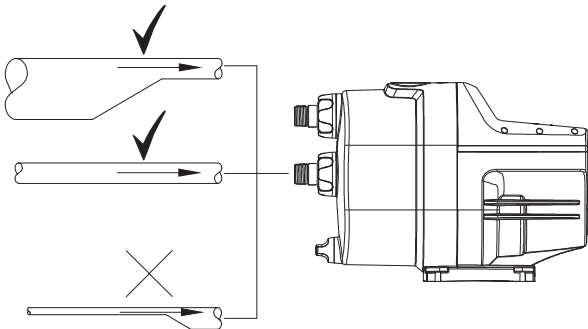
Dimensionamiento correcto de las tuberías conectadas a las conexiones de aspiración y descarga de la bomba
