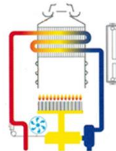
DIAGRAMA FUNCIONAL
