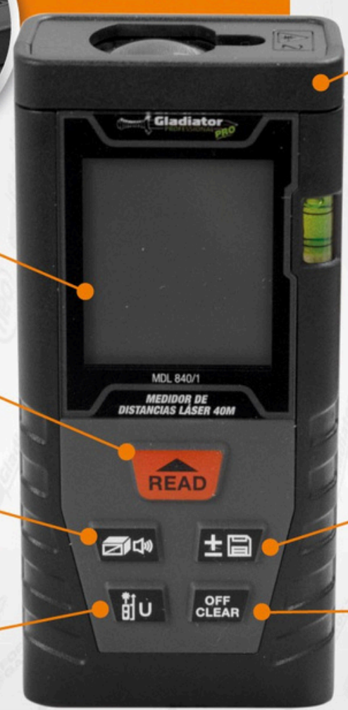
Emisor y receptor de láser
